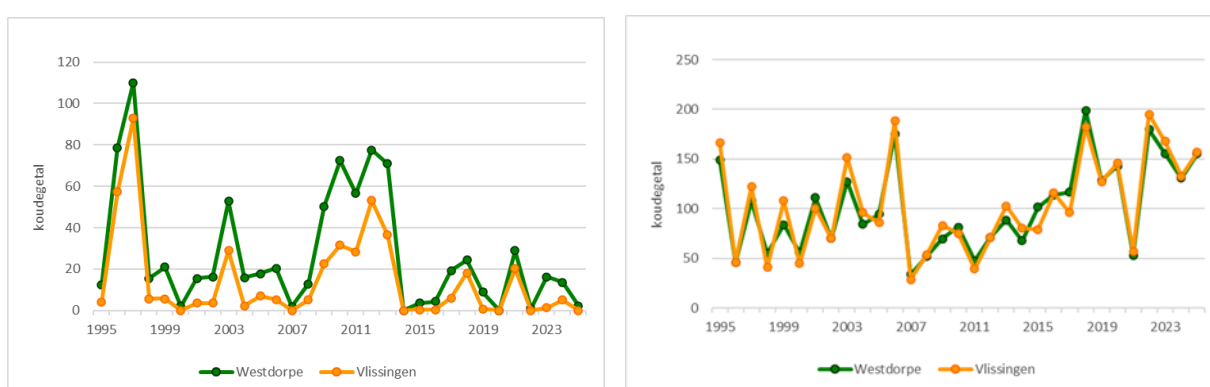
Figuur 3. Koudegetal (links) en warmtegetal (rechts) volgens Hellmann voor Vlissingen en Westdorpe voor de periode 1995-2025.
