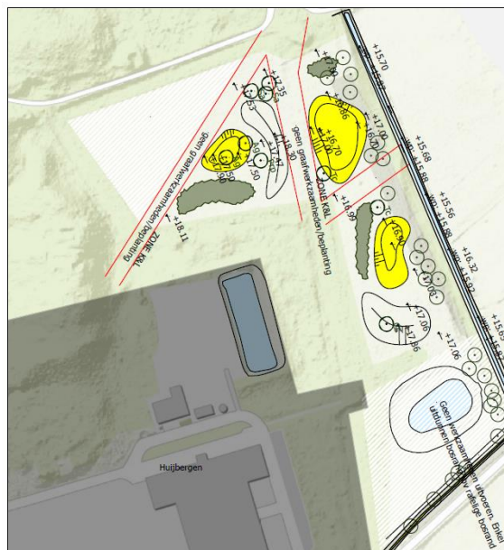
Afb. 15 Nieuwe poelen (geel) naast het pompstation
